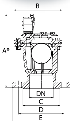
Doble Cámara Triple Acción Bridada
