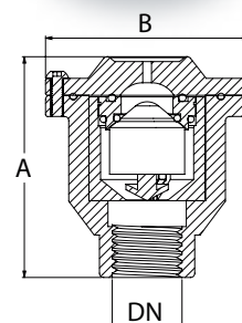
Cámara Sencilla Doble Acción Roscada
