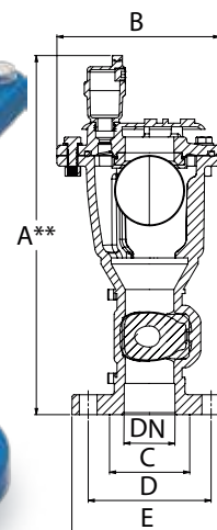
Doble Cámara Triple Acción Bridada Antifraude
