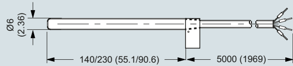
Pt500, sensor de temperatura a 4 hilos, dimensiones en mm (pulgadas)
