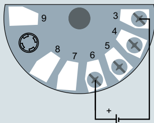
Entrada de tensión (unipolar o bipolar)
