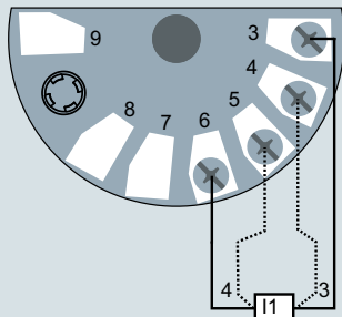
RTD a 2, 3 o 4 hilos, o resistencia lineal
