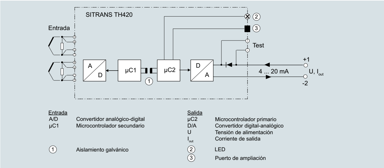
SITRANS TH420, diagrama de función
