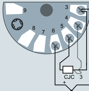
TC (CJC interna o CJC externa a 2 o 3 hilos)
