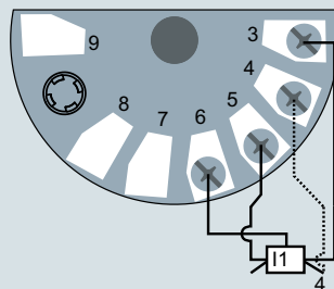
Potenciómetro a 3 o 4 hilos
