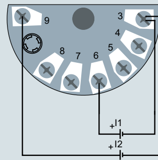
Entrada 1 o 2: Entrada de tensión (unipolar o bipolar)
