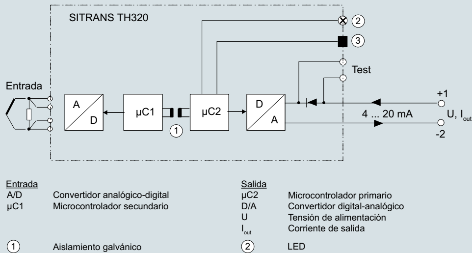
Diagrama de funciones SITRANS TH320
