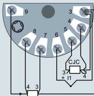
Entrada 1: TC (CJC interna o CJC externa a 2 o 3 hilos) Entrada 2: RTD a 2, 3 o 4 hilos
