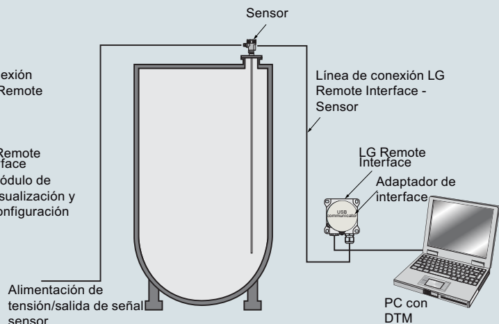
Conexión del LG Remote Interface a el sensor y el PC
