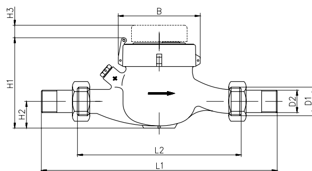
Dimensiones MTKD-N, MTKD-L-N con emisor de impulsos
